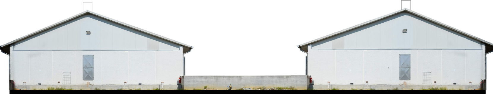
Sezione 9 1:200
