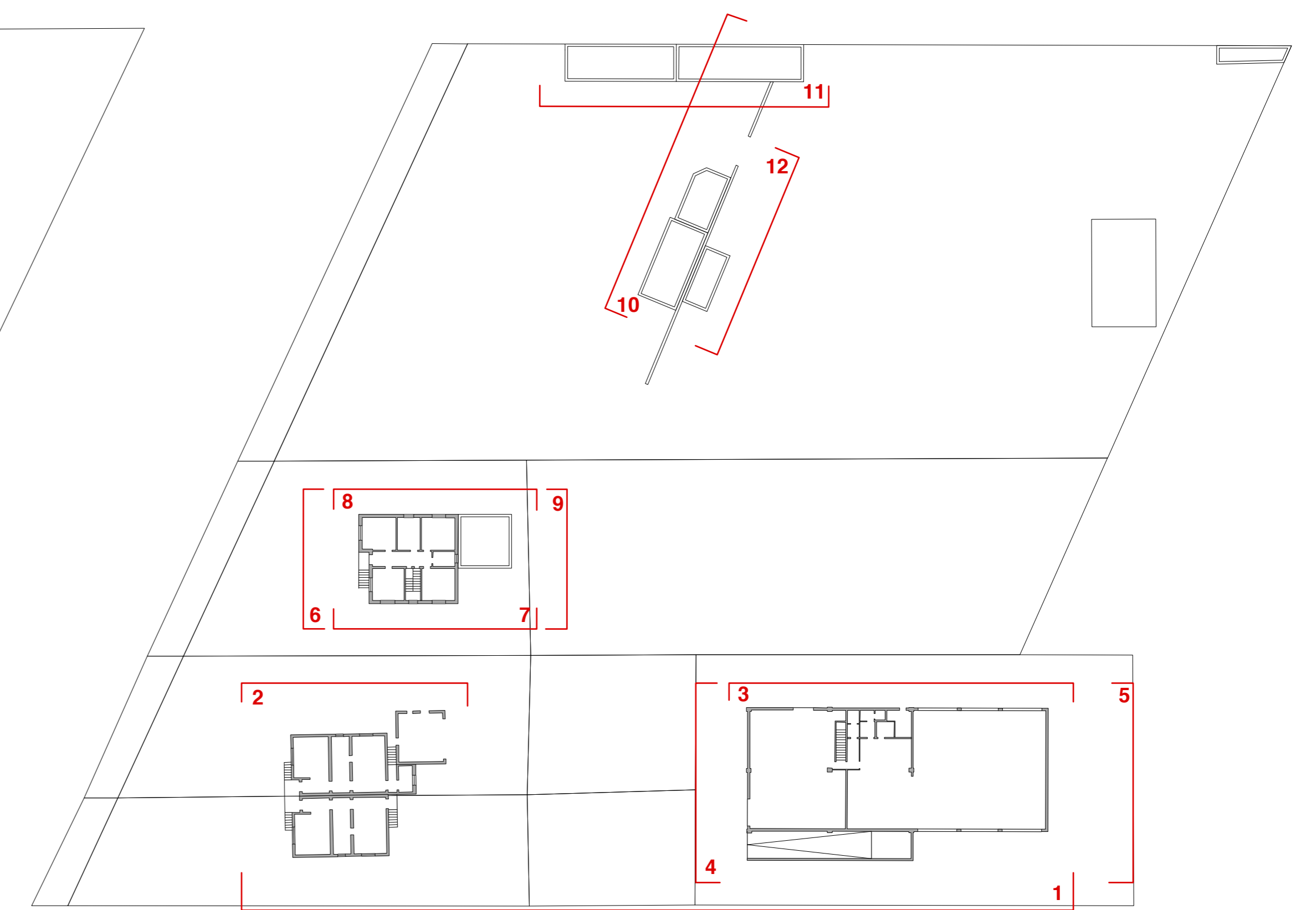
Piani terra ed individuazione sezioni 1:500
